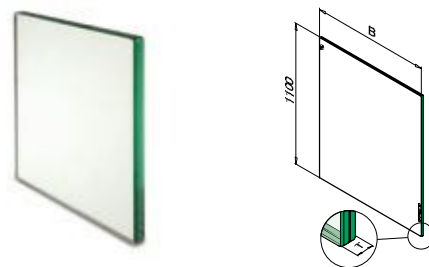
MOD 11 - VSG (2X ESG)* - H=1100 mm
