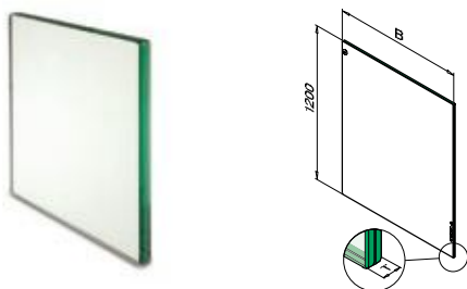
MOD 12 - VSG (2X ESG)* - H=1200 mm
