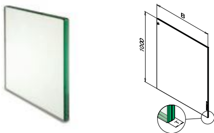
MOD 10 - VSG (2X ESG)* - H=1000 mm
